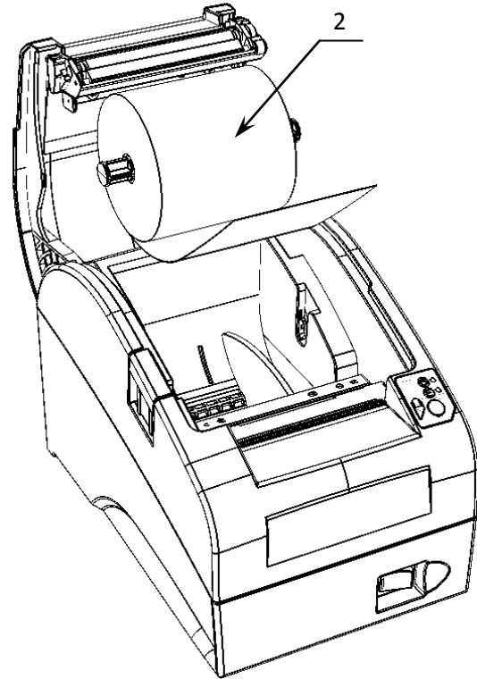
Рисунок 9. Установка ЧЛ
