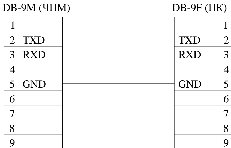
Рисунок 1 - Схема распайки кабеля подключения ЧПМ к ПК
